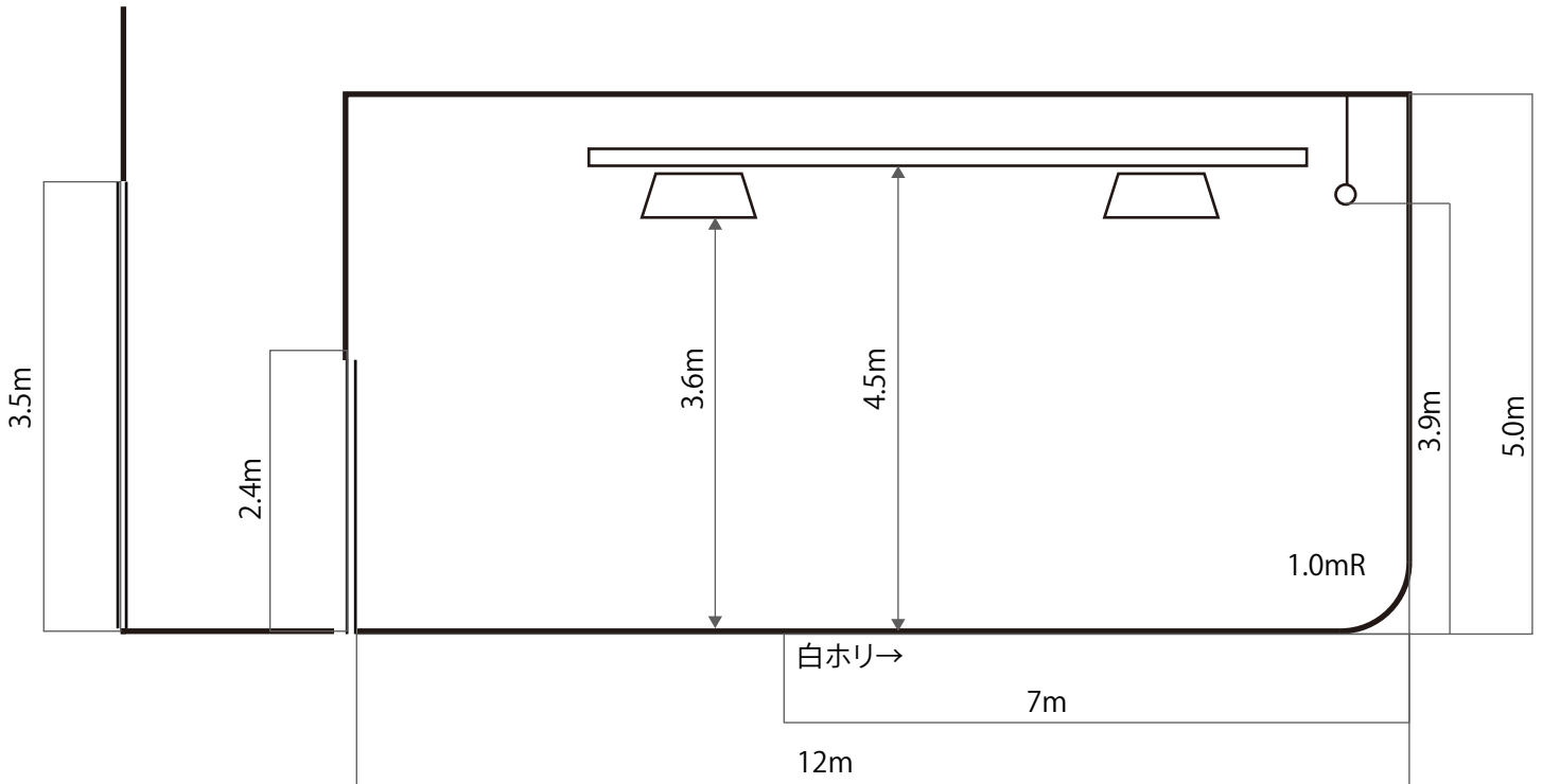
↓ 立面図
